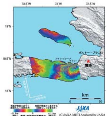
▲地震前(2009年2月28日)と地震後(2010年1月16日)のPALSARデータから得られた差分干渉画像(地殻変動図)
